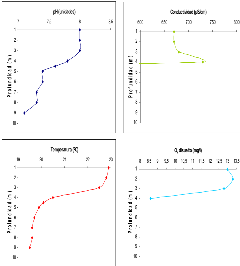
GRÁFICO 1 PERFILES FÍSICO-QUÍMICOS DEL EMBALSE
